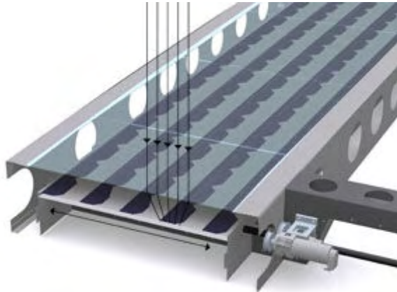
Principe van de Fresnellenzen
